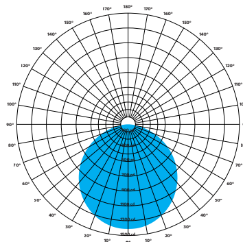
CQ2-LED1 (DIRECT)
